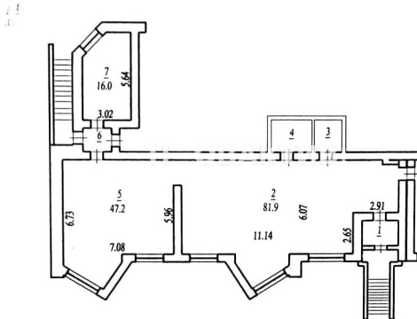
Цокольный этаж
