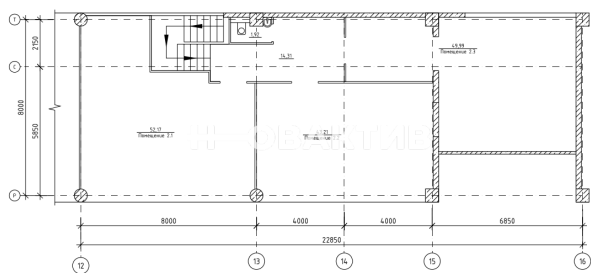
План 2-го этажа
