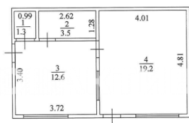
1-ый этаж
