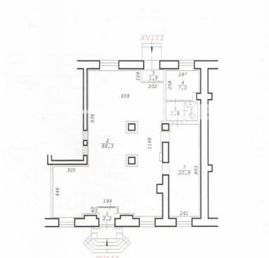
Фрагмент 1 этажа
