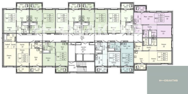
КОРПУС 1 Секция 1.1 План 6-17 этажей
